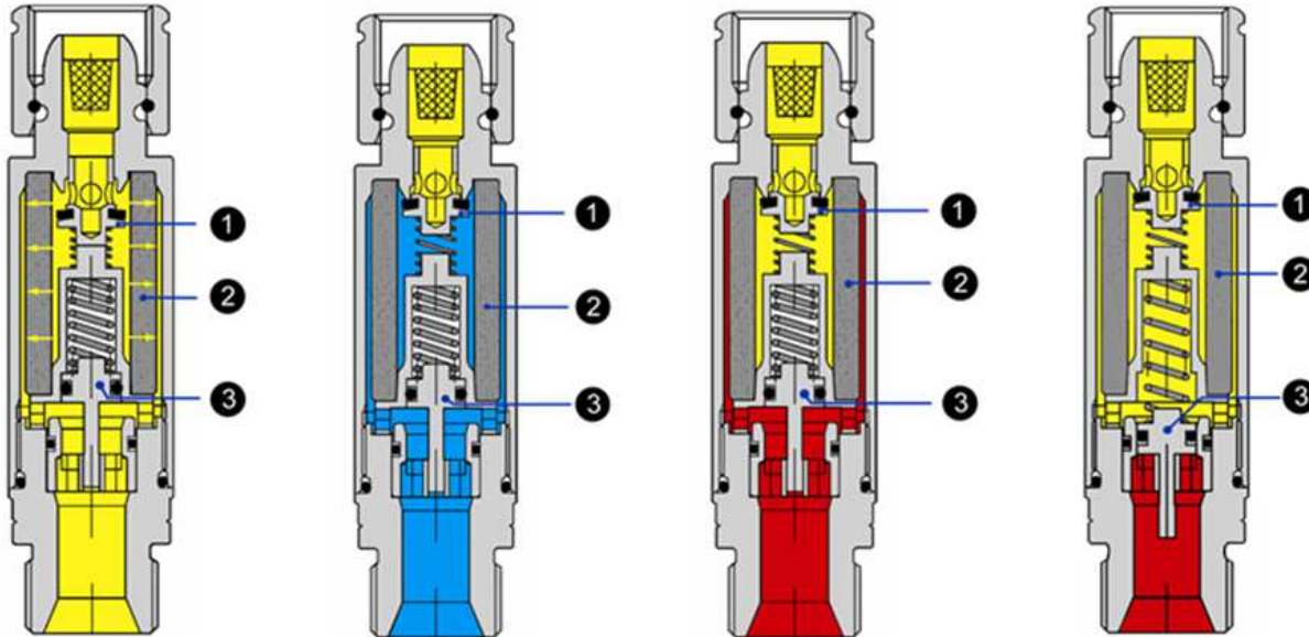
1: Gasrücktrittventil
